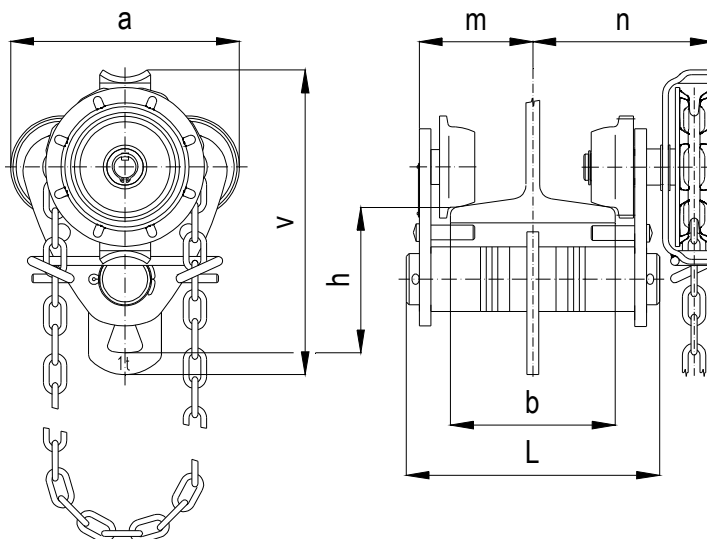
OBR. 5.1.2. MAČKY JEDNONOSNÍKOVEJ , TYP Z 410R-A, Z 410R-B nosnosť 1 t
