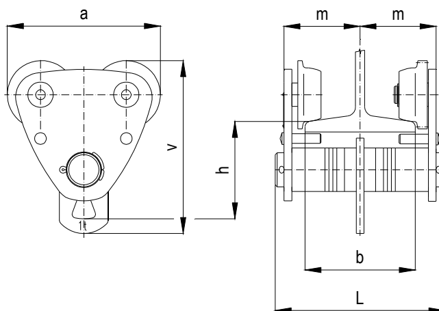
OBR. 5.1.2. MAČKY JEDNONOSNÍKOVEJ , TYP Z 410R-A, Z 410R-B nosnosť 1 t
